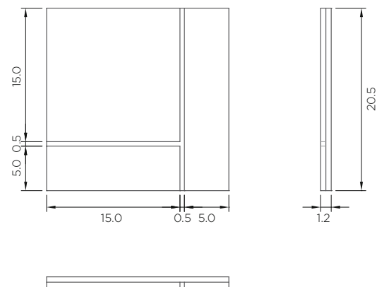
PVC ou MDF vistas ortográficas
