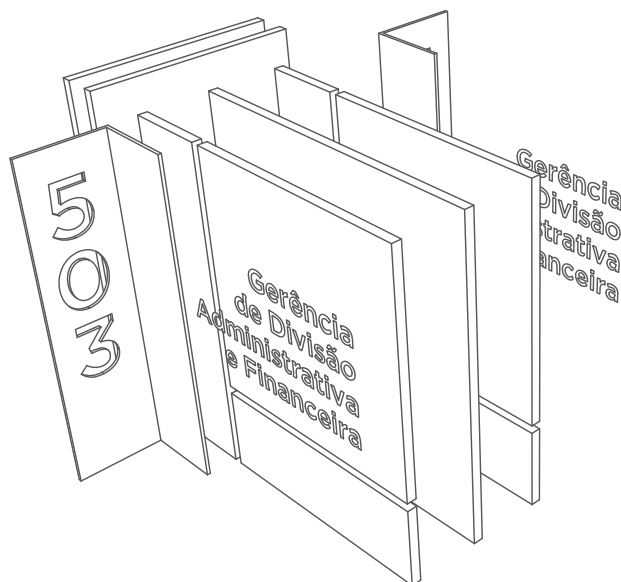
Peças completas vista explodida
