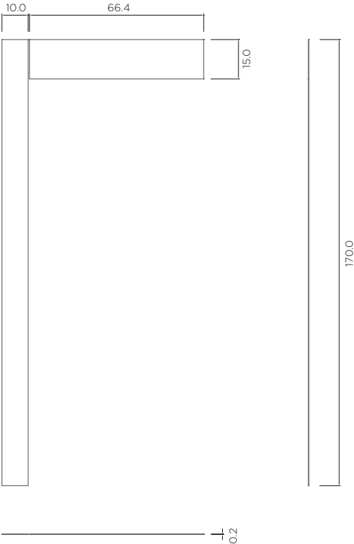
Chapa de acrílico e textos vistas ortográficas
