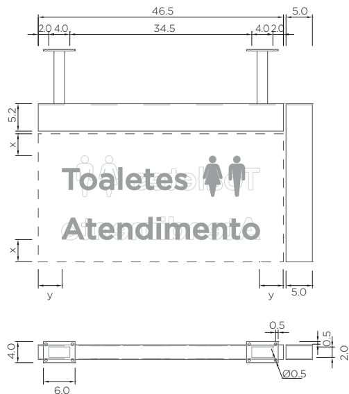
Chapa metálica e textos vistas ortográficas
