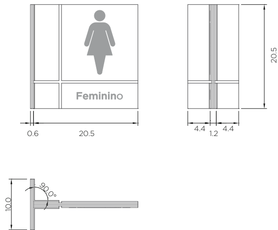
Peças montadas vistas ortográficas
