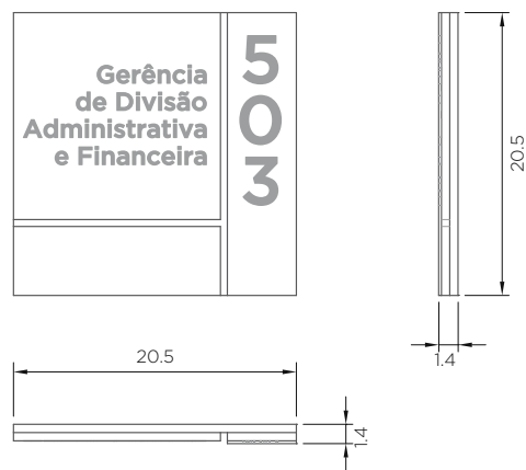
Peças montadas vistas ortográficas
